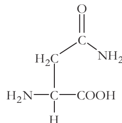
Asparagine
